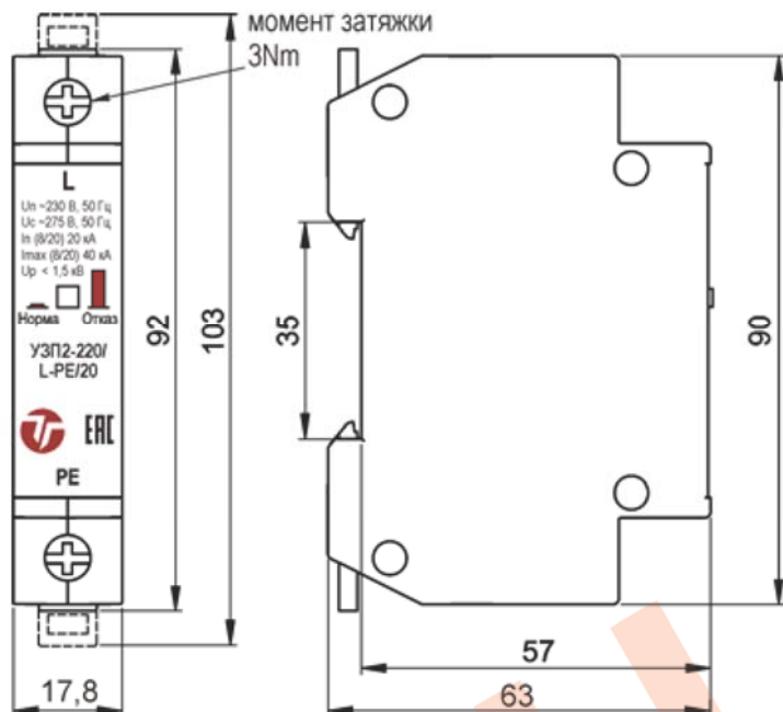
Рис.1 Габаритные размеры
